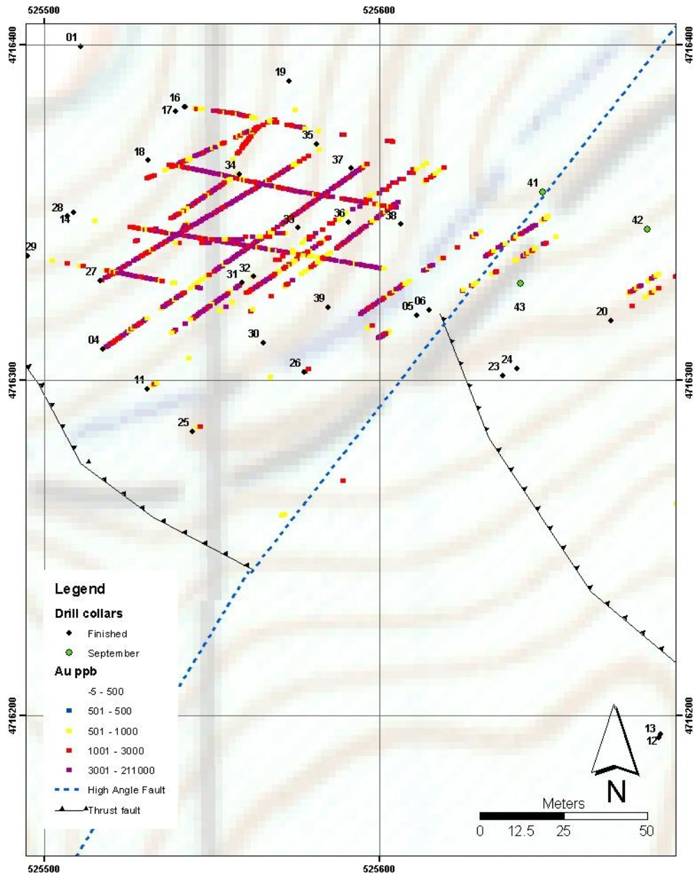
Abbildung 2. In den Bohrungen bis SLV036 durchteufte Goldmineralisierung in den Zonen Peshter Gossan und Extension.
